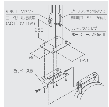
取付参考図
